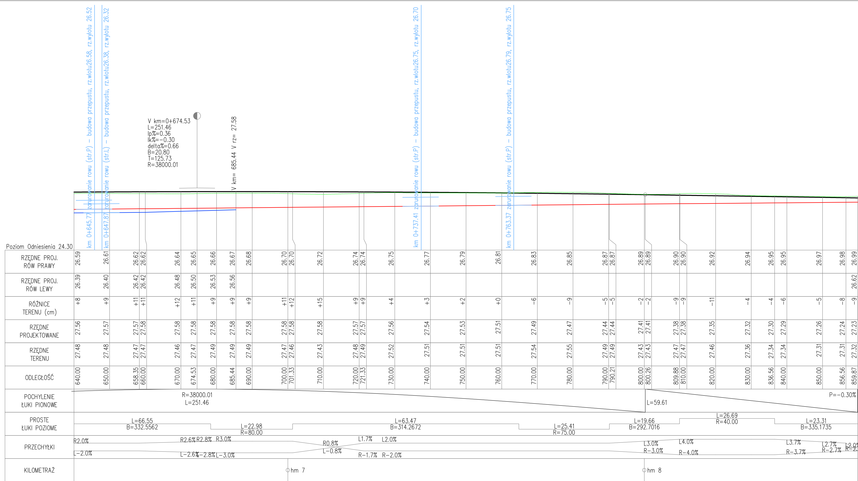
PROFIL PODŁUŻNY DR GMINNA Pocztek trasy km: 640.000 Koniec trasy km: 859.871 SKALA Pozioma 1:500 Pionowa 1:100
